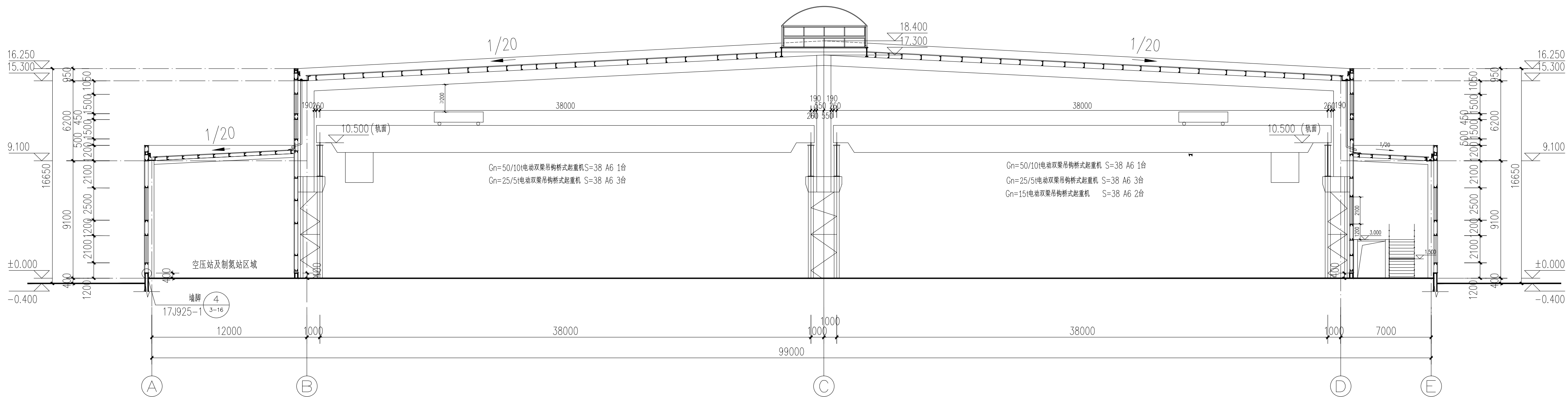
1-1剖面图 1:200
